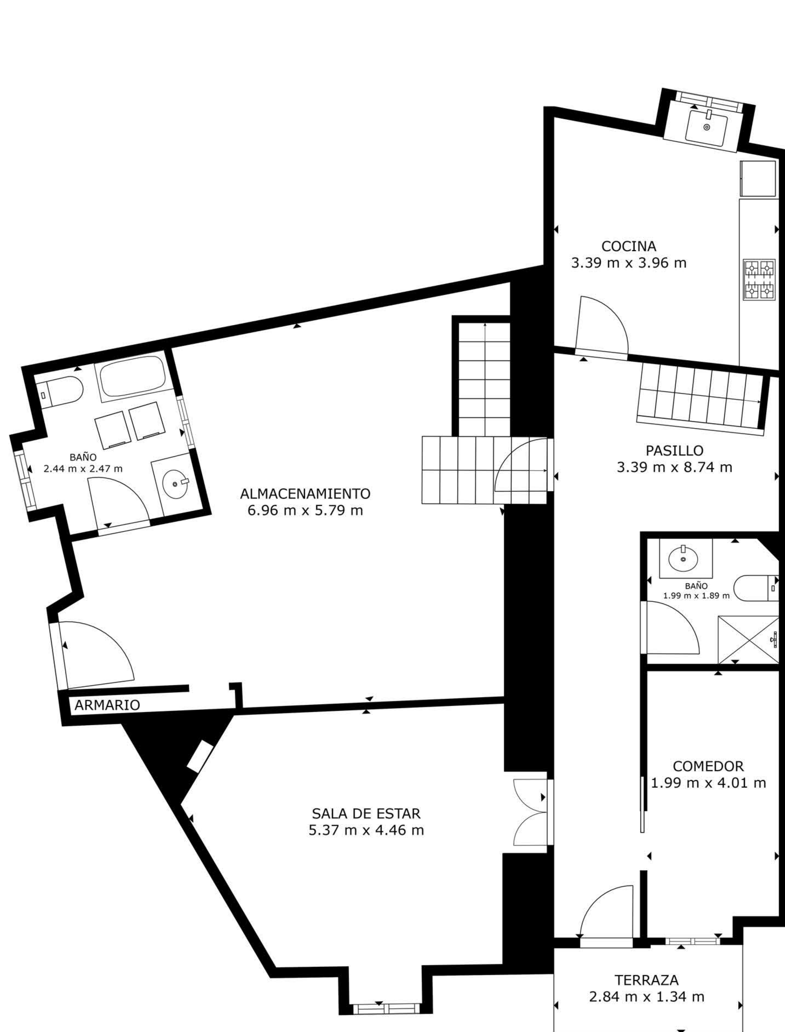
PLANTA 1
