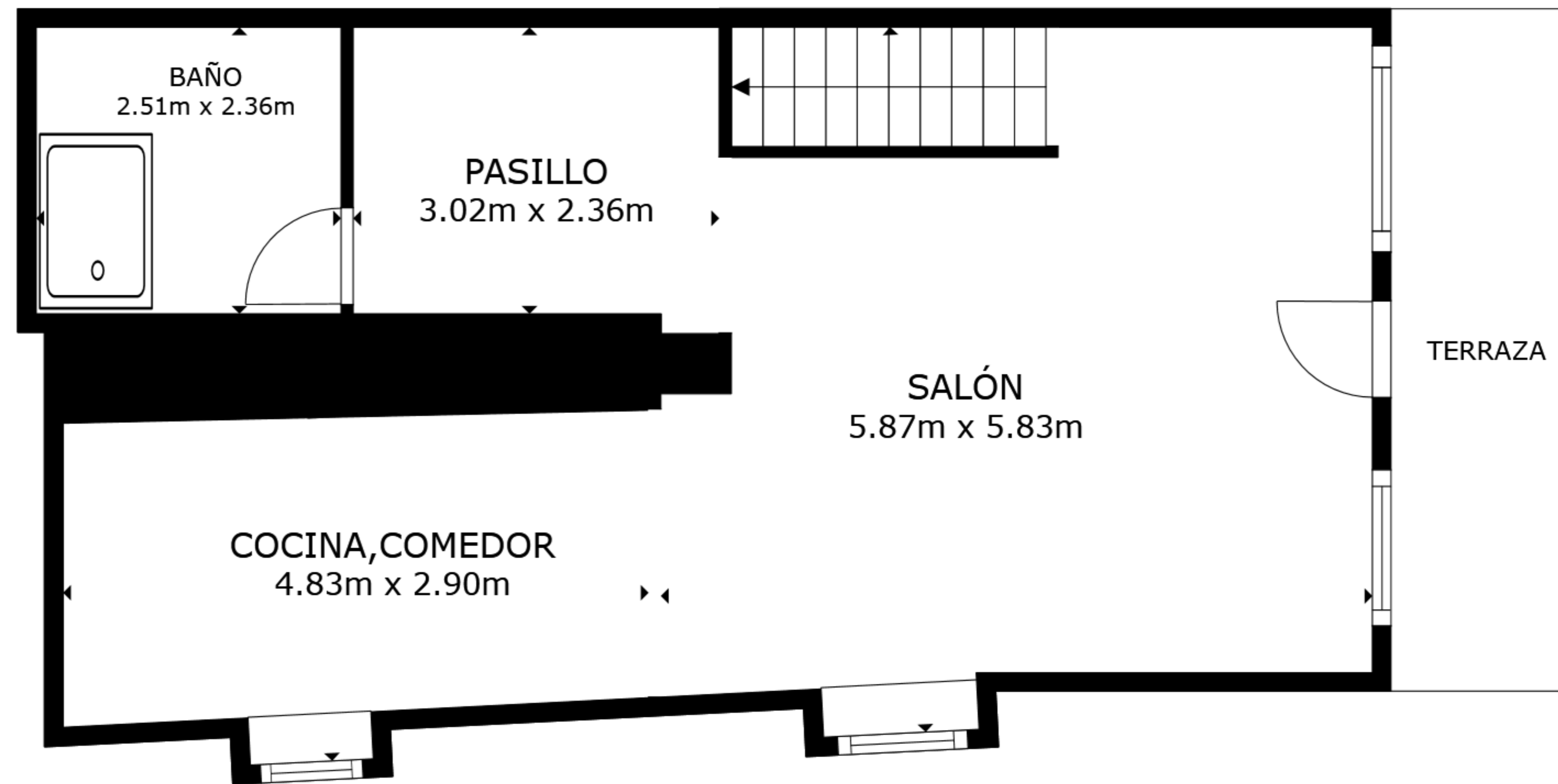
PLANTA 1
